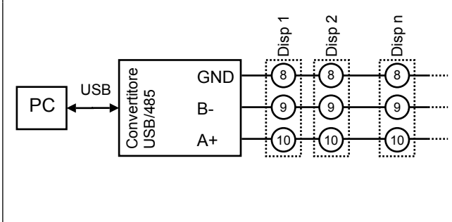
Comunicazione su morsetto estraibile 8-9-10 configurato in modalità RS485
