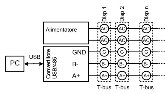
Comunicazione su connettore T-Bus (richiede l'accessorio opzionale)
