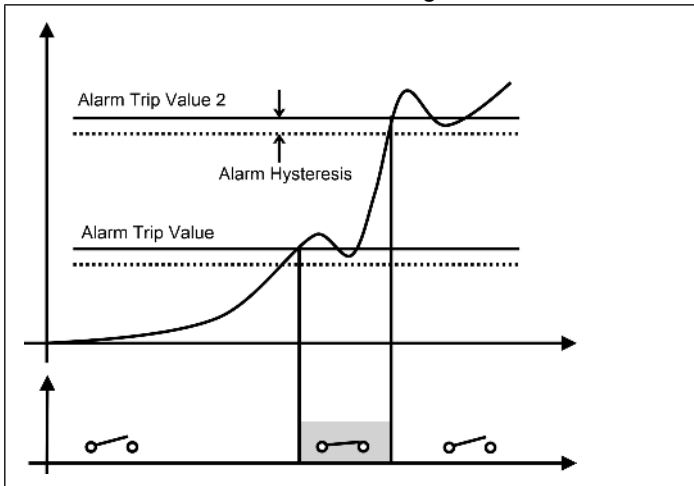
A finestra: contatto chiuso tra le soglie
