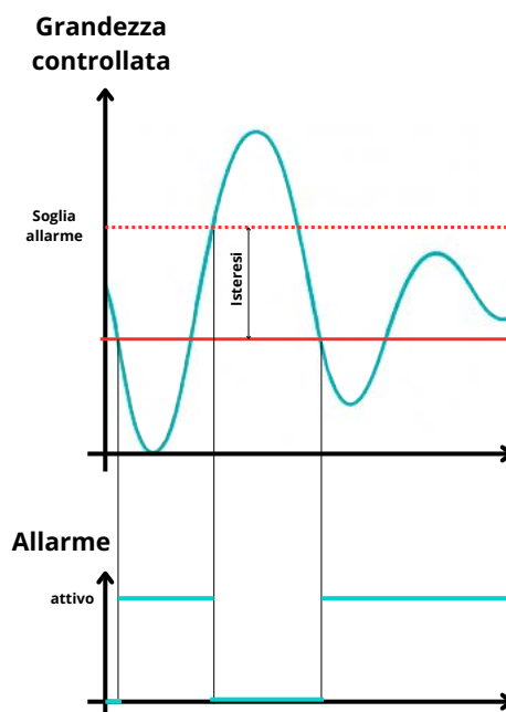
Figura 4: Allarme sotto soglia
