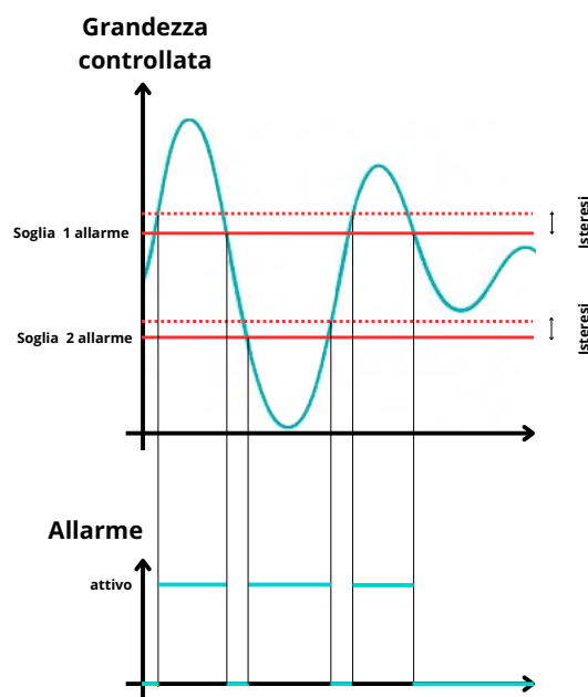
Figura 6: Allarme fuori dalle soglie
