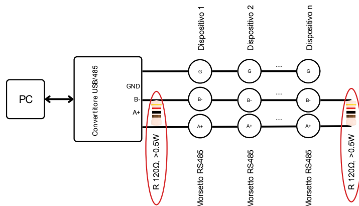
Figura 2: Terminazione bus RS485
