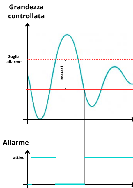
Figura 5: Allarme sotto soglia
