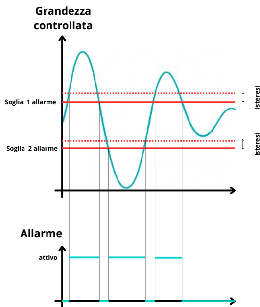
Figura 7: Allarme fuori dalle soglie
