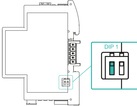
Figura 11: Dip-switch per configurazione baudrate
