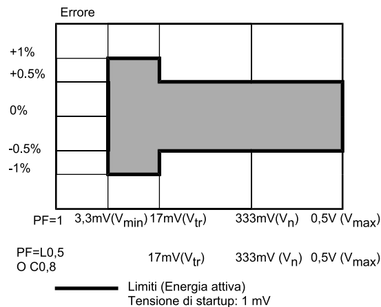
Figura 8: Wh, precisione in funzione del carico (TA con uscita in tensione)
