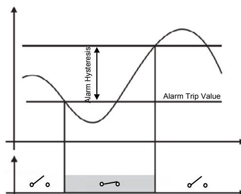
Figura 4: In discesa: contatto normalmente chiuso
