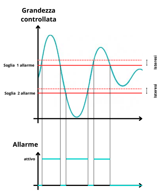
Figura 7: Allarme fuori dalle soglie
