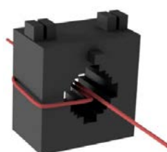
2 spire (2 passaggi attraverso il nucleo)
