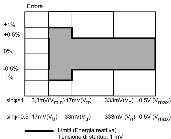
Figura 11: VARh, precisione in funzione del carico (TA con uscita in tensione)
