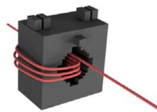
4 spire (4 passaggi attraverso il nucleo)
