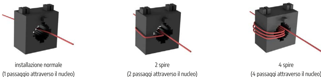
Figura 1: esempi di avvolgimenti
